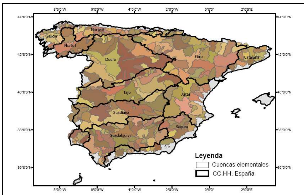
Figura I.- Cuenca elementales de estudio y cuencas acumuladas (cuencas hidrográficas de la planificación hidrológica en España)
