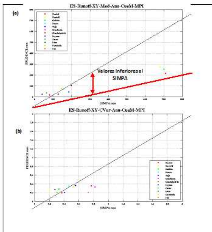
Figura V.- Contraste entre datos observados (SIMPA) y simulados (PRUDENCE) en las diferentes cuencas hidrográficas de la planificación hidrológica de España: (a) escorrentía media anual y (b) coeficiente de variación anual
